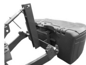
Montage avec triangle simple
