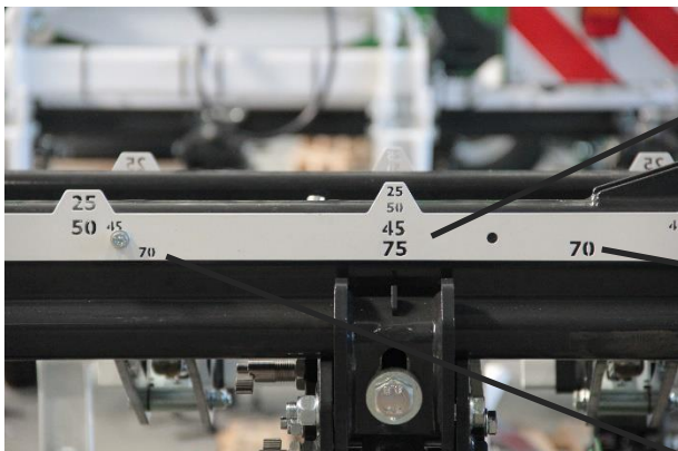
Abbildung 6: Reihenweitenskala
