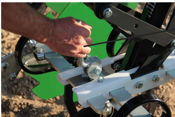
Abbildung 13: Arretierung und Positionsraster
