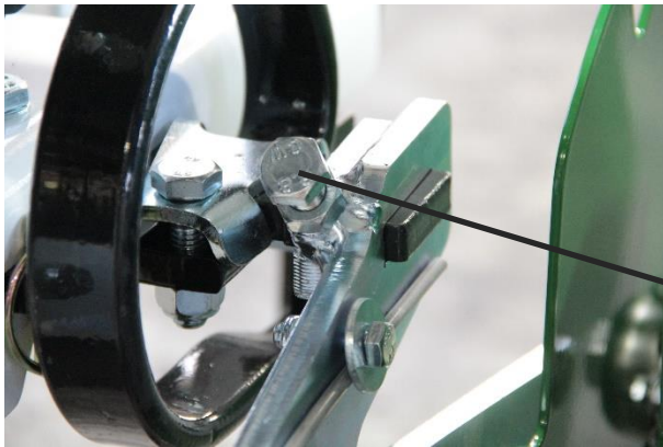
Abbildung 28: Scheibenmontage
