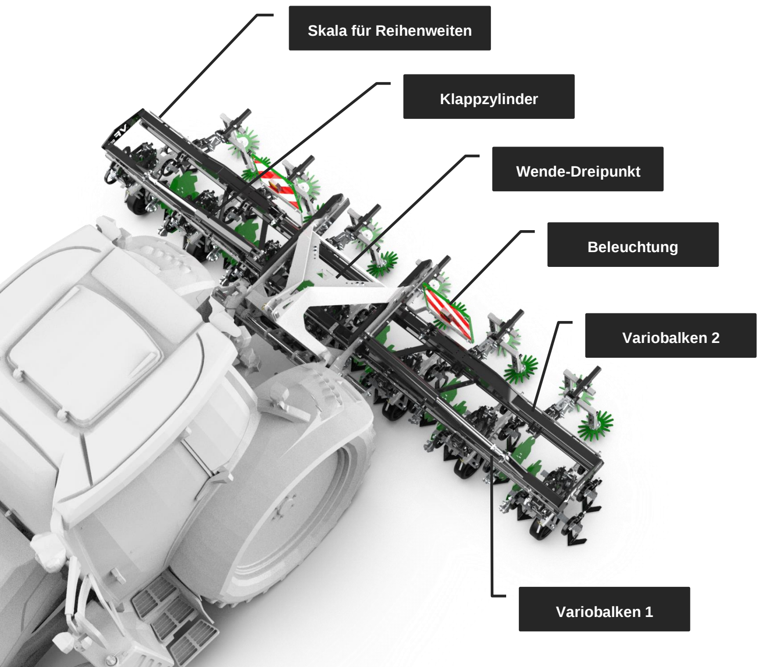
Abbildung 1: Aufbau Variofield
