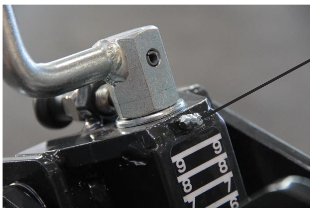
Abbildung 43: Tastradspindel
