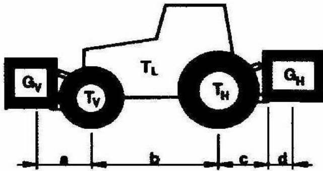
Abbildung 39: Schaubild Gewichtsverteilung
