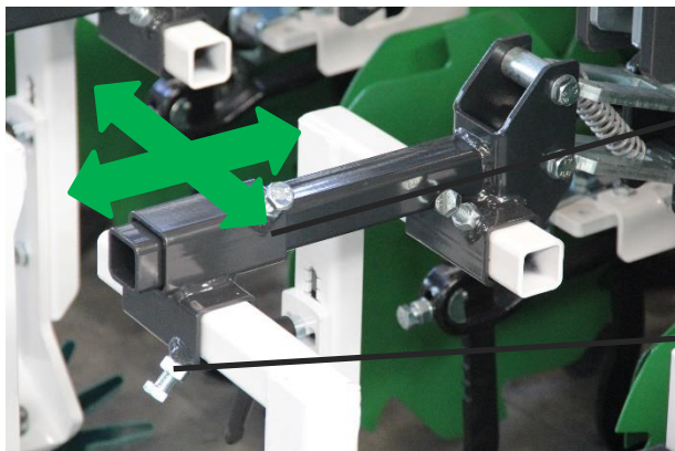
Abbildung 31: Fingerhackenträger
