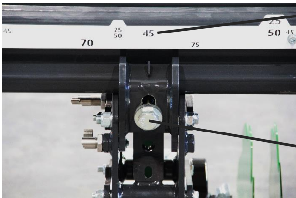
Abbildung 8: Modulklemme am Variobalken
