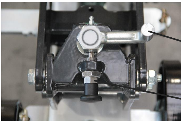
Abbildung 16: Kurbel und Verdrehsicherung
