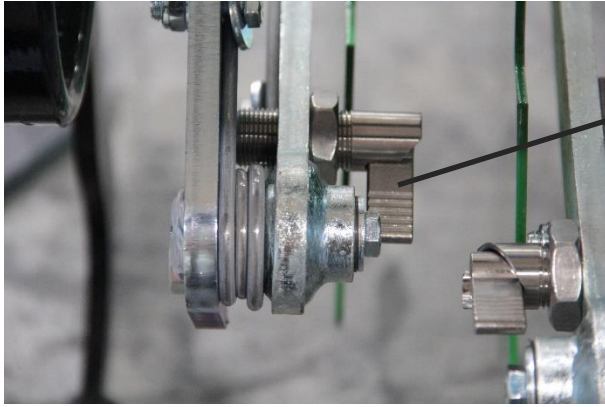
Abbildung 27: Scheibengelenk
