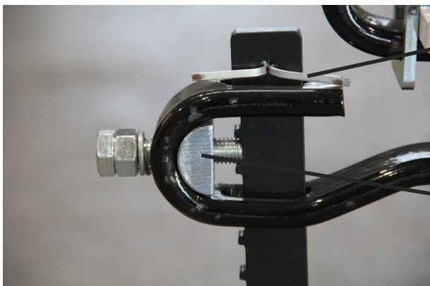
Abbildung 19: Stielklemmung
