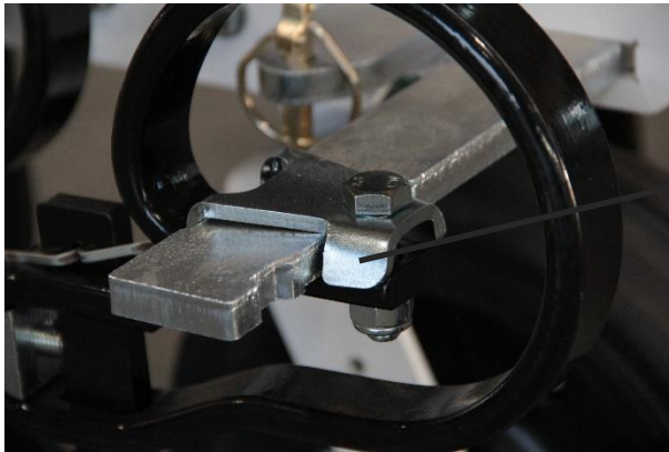
Abbildung 20: Federzinkenklemmung
