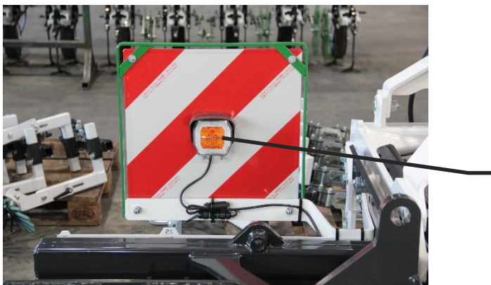
Abbildung 35: Frontbeleuchtung
