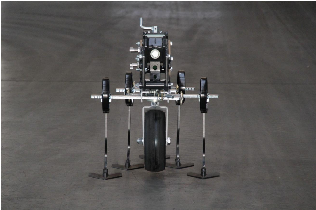
Abbildung 7: Hackmodul
