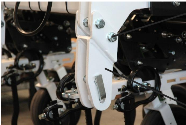
Abbildung 5: Unterlenkeranhangung
