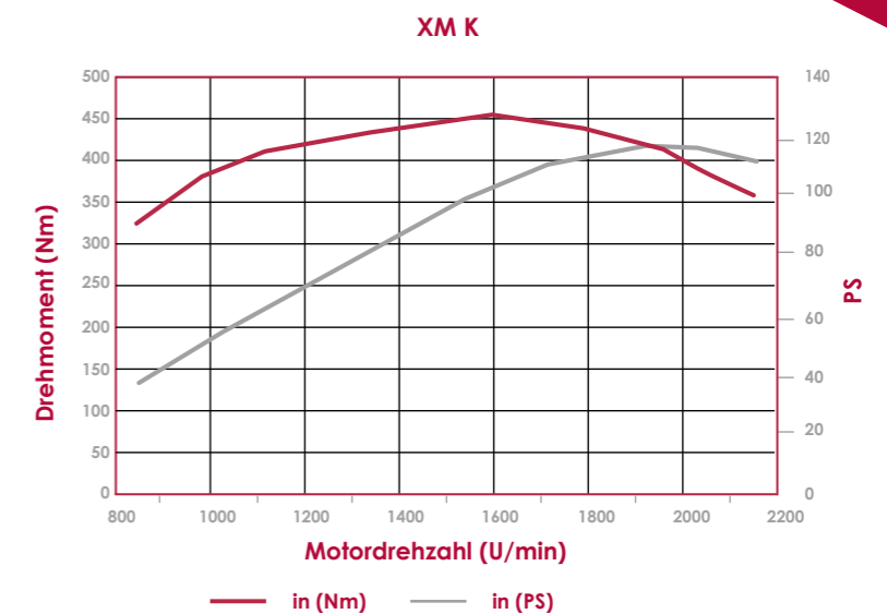
Drehmoment-/Leistungskurve Modell 120.
